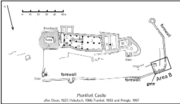
איור 1 - תכנית כללית של המבצר ובה מודגש אזור החפירה
