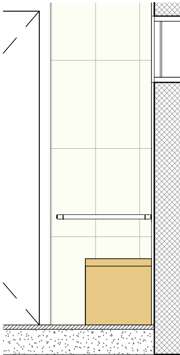
חזית 5-5 1 : 25
