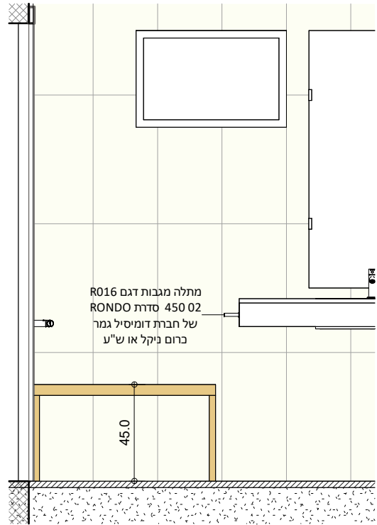
חזית 4-4 1 : 25
