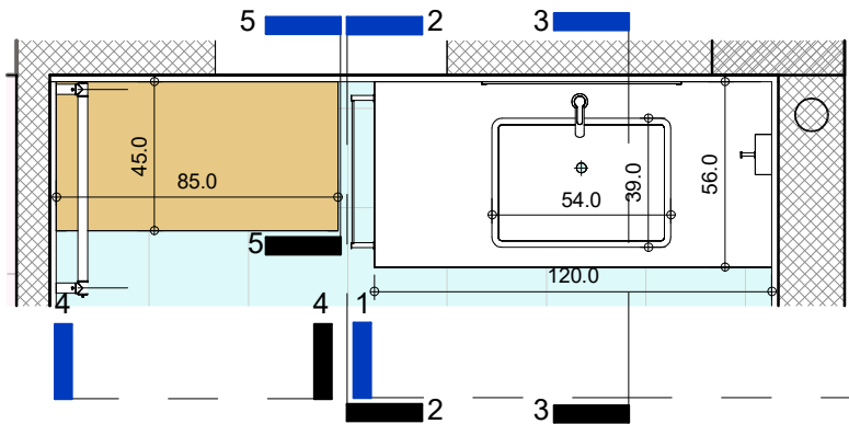
תכנית משטח לכיור וספסל הלבשה 1 : 25
