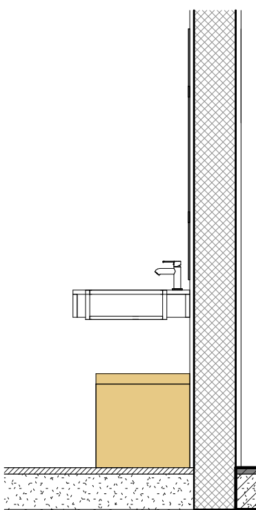
חזית 3-3 1 : 25
