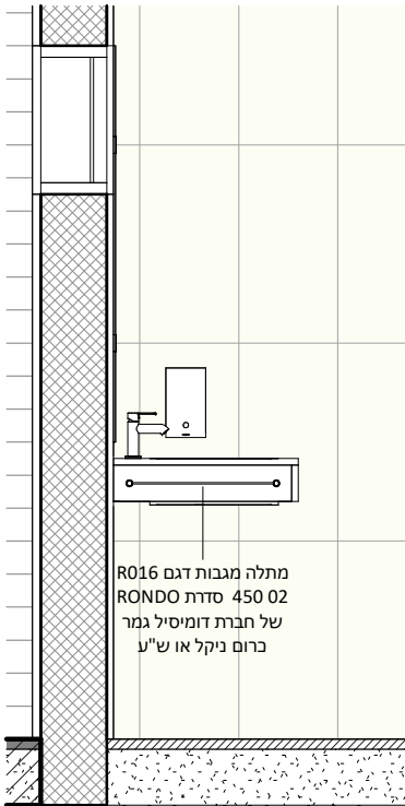
חזית 2-2 1 : 25
